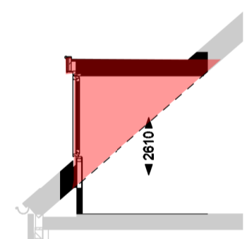
Doorsnede
