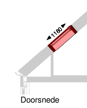
Doorsnede
