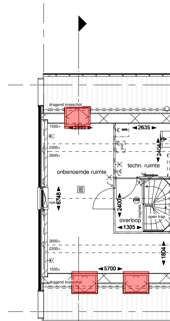
Tweede verdieping
