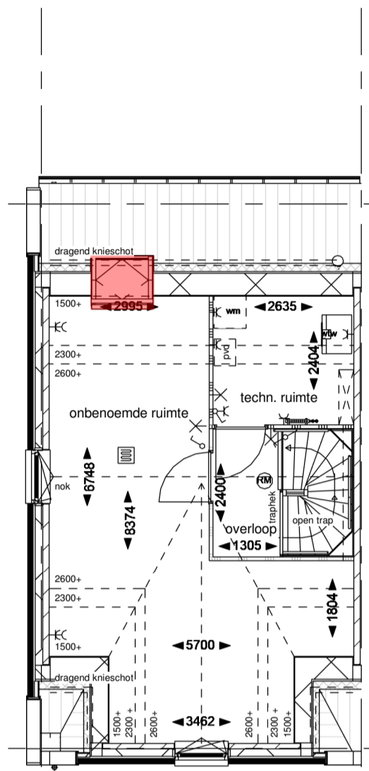
Tweede verdieping
