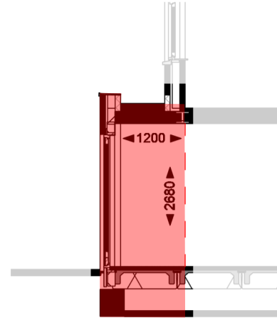
Doorsnede
